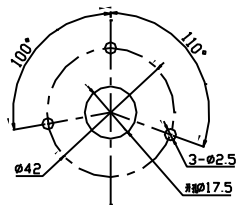
H2N/H4N 法兰安装开孔
