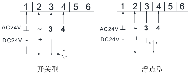
端子接线图
